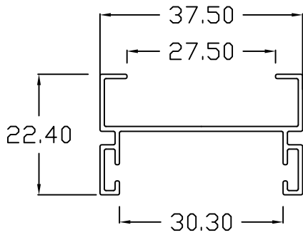
SD - 106 ASTRAGAL
