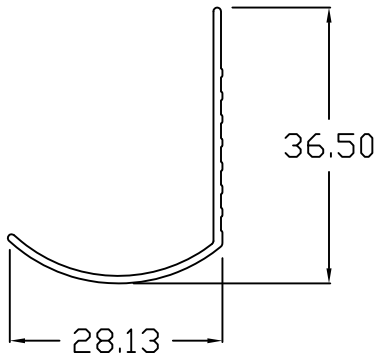
ASN 1 1/4 Stairnoising
