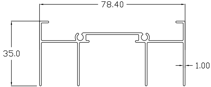
90001 HEADER
