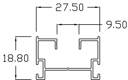
SD - 135 FIXED STILE
