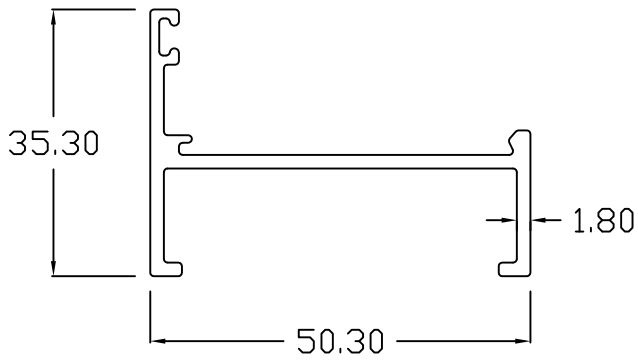
LYC - 2A
