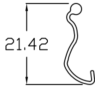
BLADE 2
