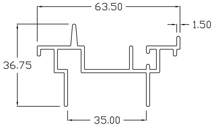
STUD
