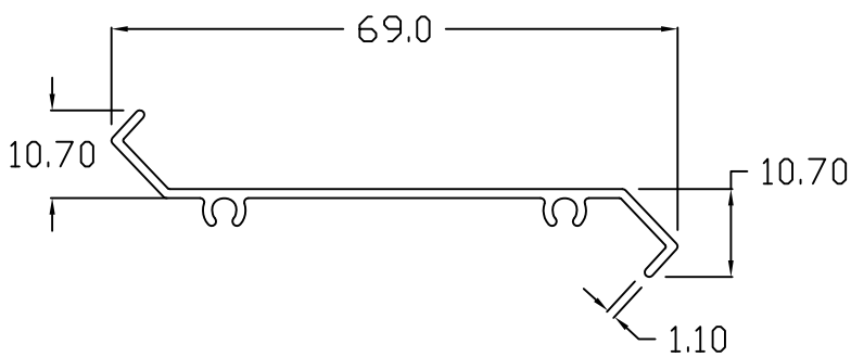
LOUVER
