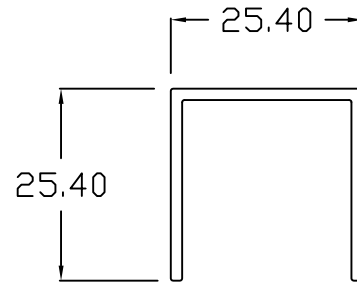
UC - 1 x 1
