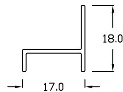
ASW - 23 SCREEN HEAD JAMB
