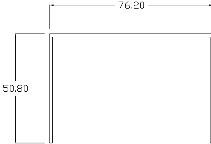
UC - 2 x 3
