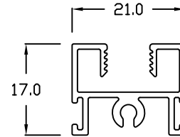
ASW - 5 TOP RAIL
