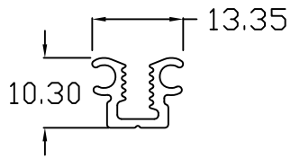
BLADE 1
