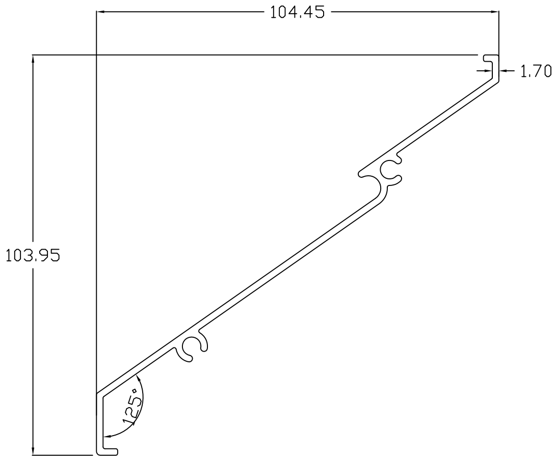
HVA 019
