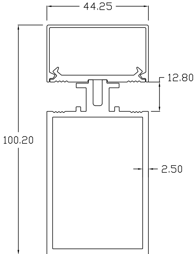
MINI MULLION WITH PIN
