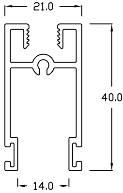
ASW - 4 BOTTOM RAIL
