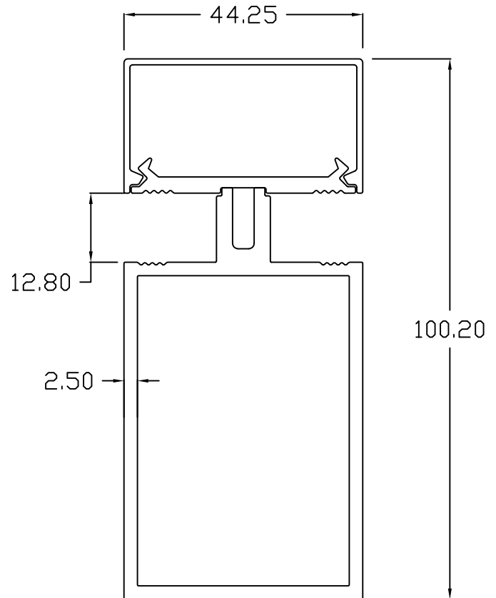
MINI MULLION STRAIGHT PIN
