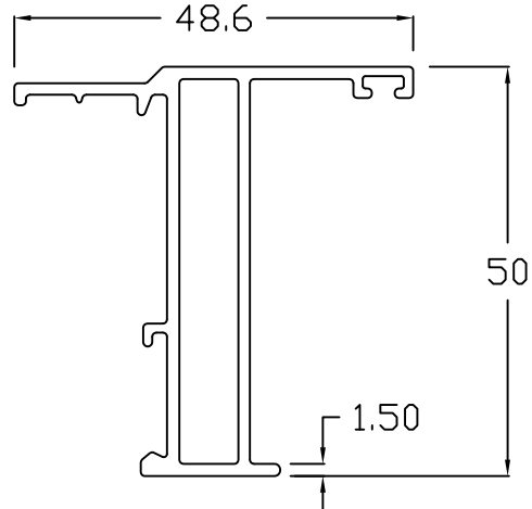
LYC - 2
