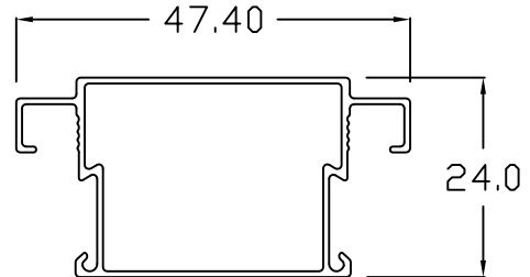
SF - 106 SC. DOOR CROSSBAR
