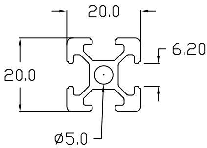
20 x 20
