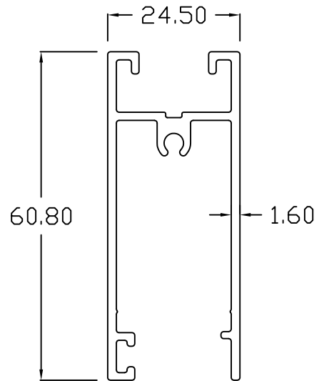
SENZA - 824 BOTTOM RAIL
