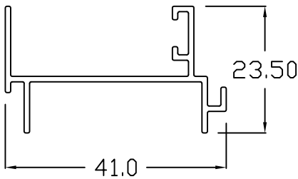
SD - 142 SINGLE JAMB
