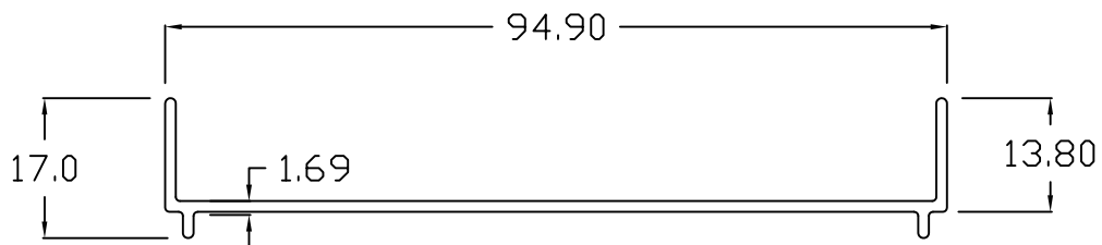
HVA S12
