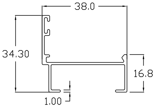
38 - 2A ( PERIMETER )
