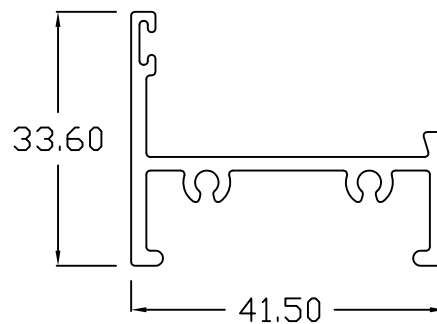
CLEO 50
