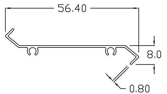
LOUVER
