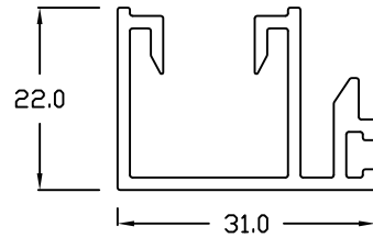
ASW - 17 INTERLOCKER
