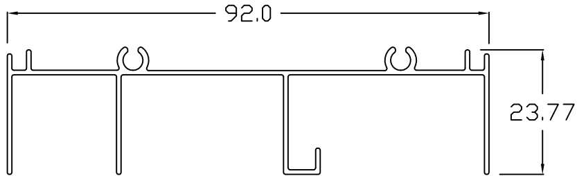
SD - 146
