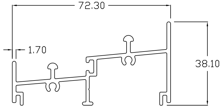
SENZA - 831 DOUBLE SILL
