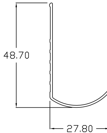
ASN 1 3/4 Stairnoising
