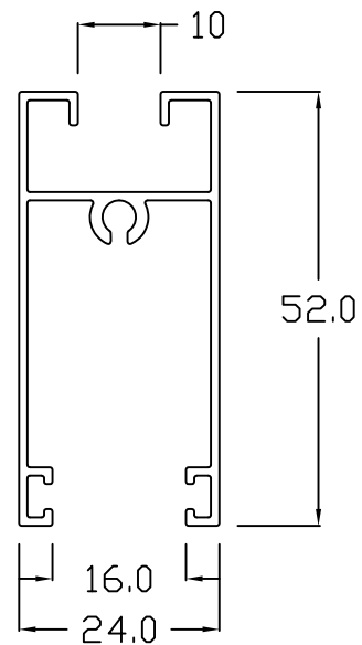
SD - 204
