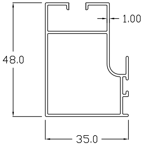
90007 INTERLOCKER
