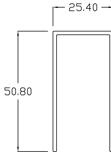
UC - 2 x 1
