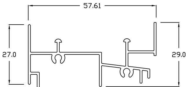
ASW - 13 DOUBLE SILL
