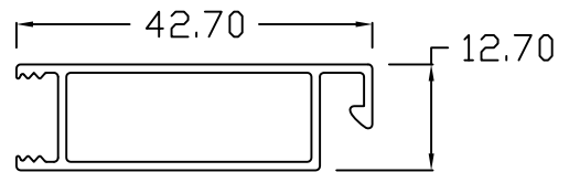
YS - 221 SCREEN FRAME
