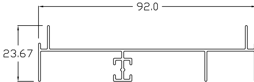
SD - 147
