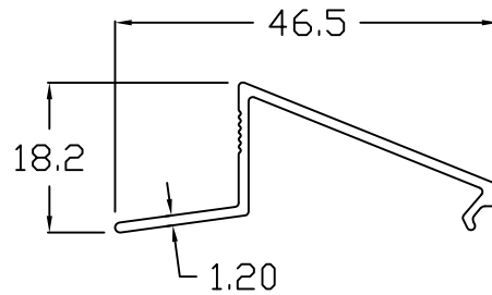
LYC - 12
