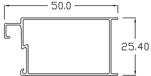
SF - 101 SCREEN DOOR FRAME
