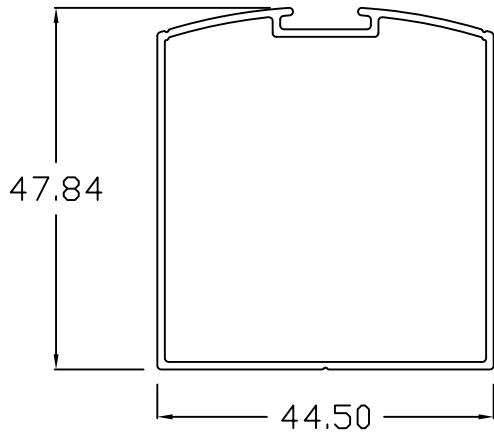
ED - 103 STILE W/ GROOVE
