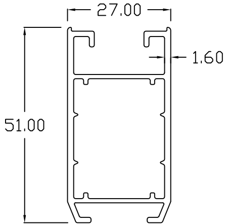
SENZA - 803 LOCKSTILE
