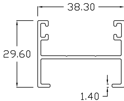
SENZA - 806 ASTRAGAL
