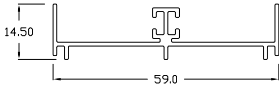
ASW - 15 DOUBLE JAMB
