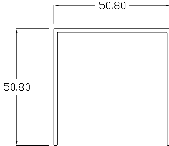
UC - 2 x 2
