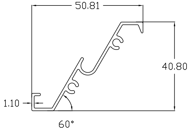
HVA 252
