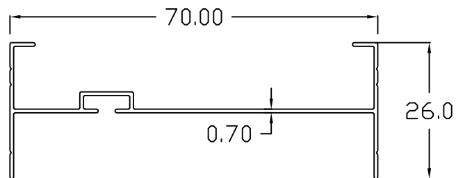
DOUBLE JAMB
