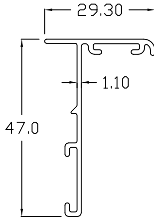
SLOT FRAME
