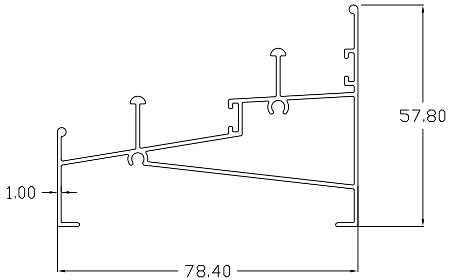
90002 SILL
