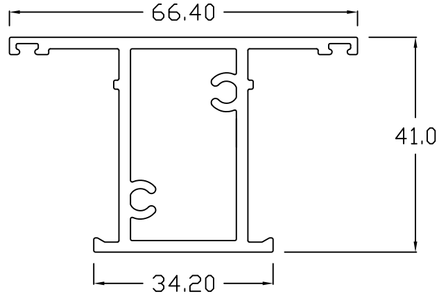
CLEO 48
