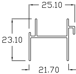
SD - 140 SCREEN JAMB
