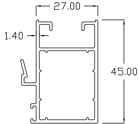
SENZA - 805 INTER LOCKER
