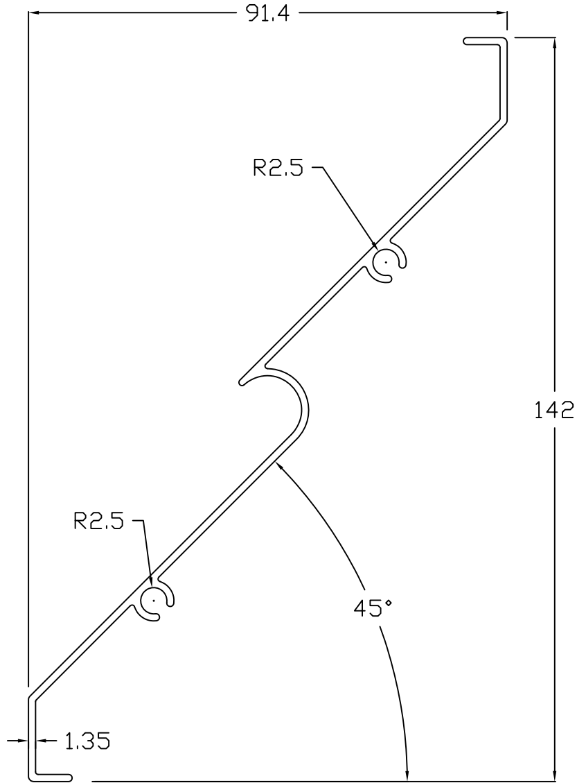
HVA S11
