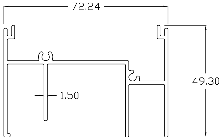
SENZA - 832 DOOR HEAD
