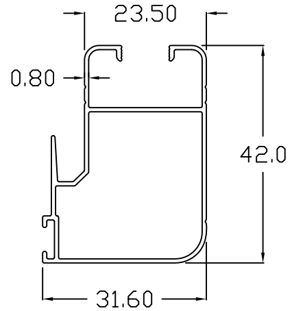
INTERLOCKER
