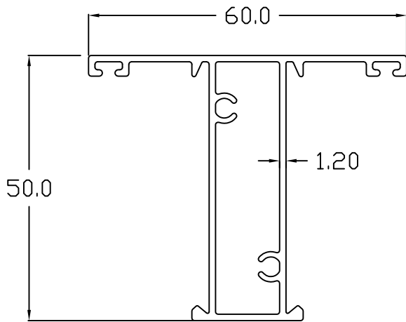
50 - 4
