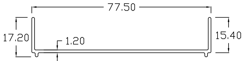
WVA - 43
