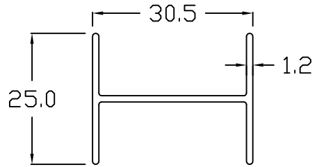
9000 ASTRAGAL
