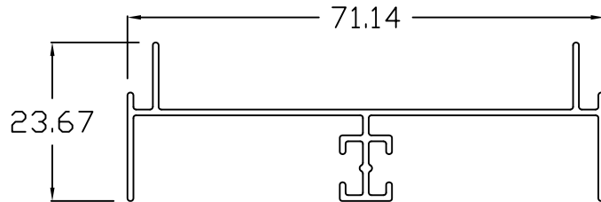
SD - 134 DOUBLE JAMB
