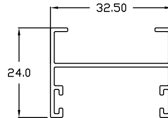
ASW - 8 ASTRAGAL
