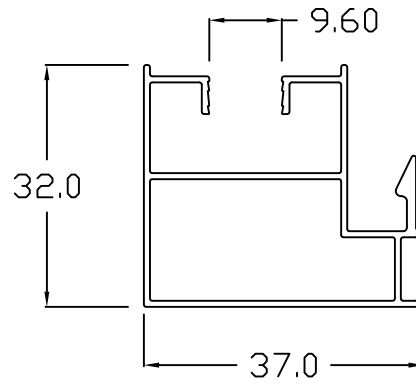
SD - 104 INTERLOCKER
