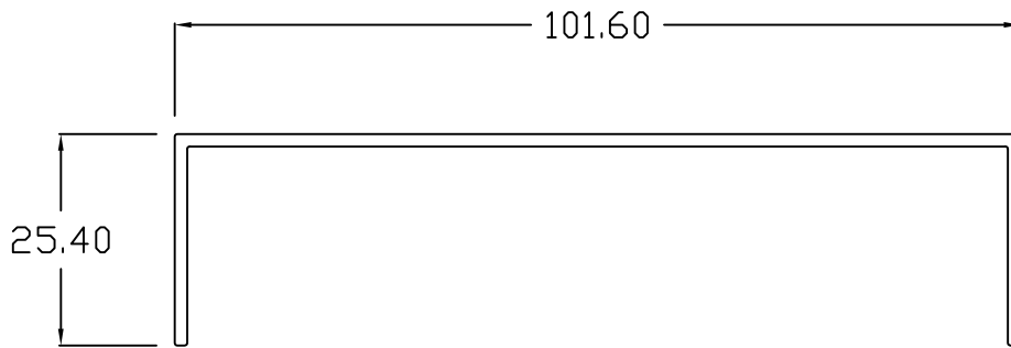
UC - 1 1/2 x 4
