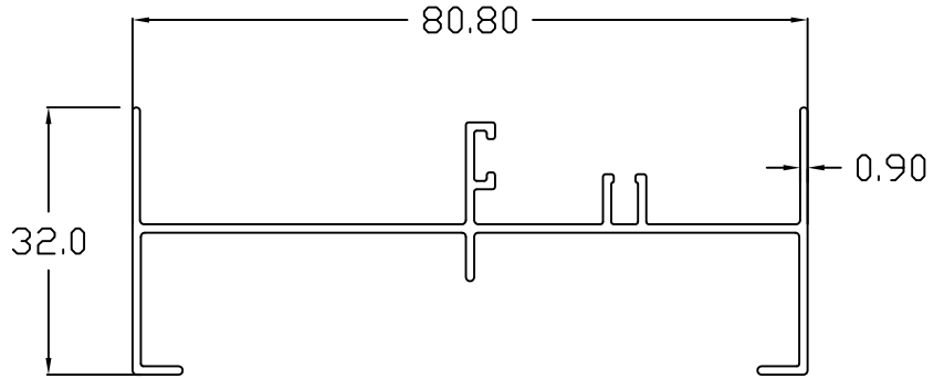
90003 JAMB
